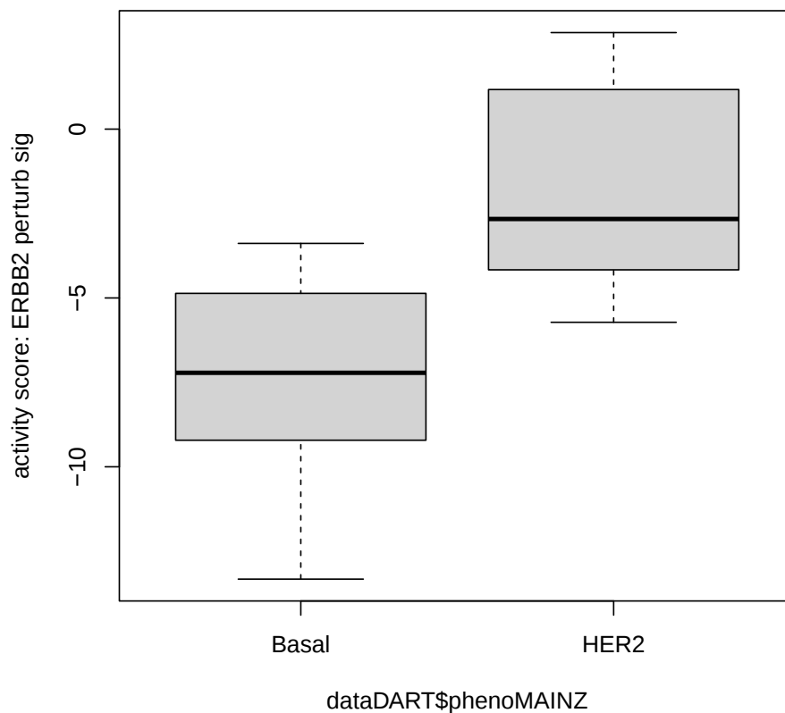
DoDART – Mainz data set: P=0.00019
